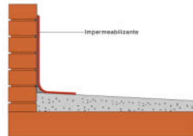
Aplicación capa adherencia de refuerzo
