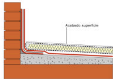
Terminación de superficie según proyecto
