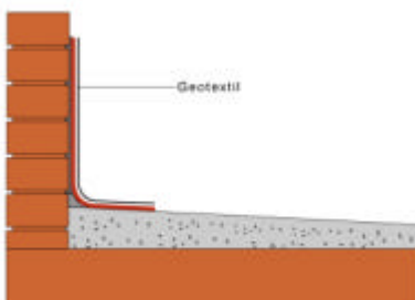
Colocación malla refuerzo
