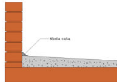
Confección de la media caña
