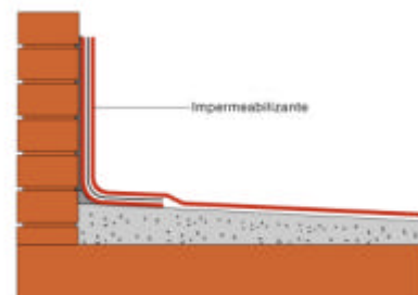
Aplicación de impermeabilizante según consumos y metros 2 indicados en las fichas técnicas.
