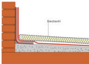
Colocación de geotextil de separación
