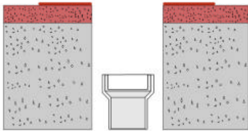
Capa de impermeabilización para adherencia cazoleta.
