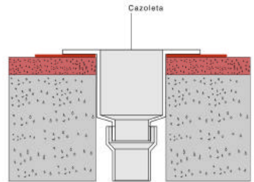
Colocación de cazoleta prefabricada.
