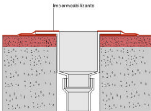
Impermeabilización general de la superficie reforzando perímetro de la cazoleta.
